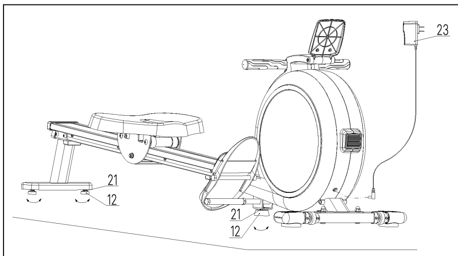
Рисунок 7 – Готовая сборка тренажера
