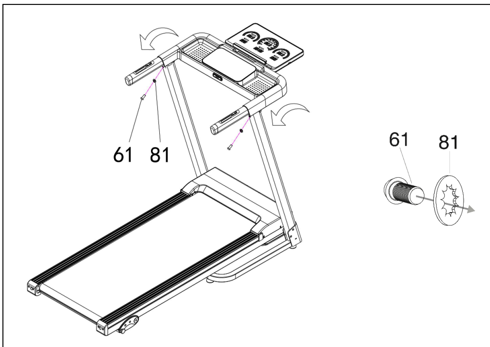
Рисунок 3 — Установка консоли беговой дорожки
