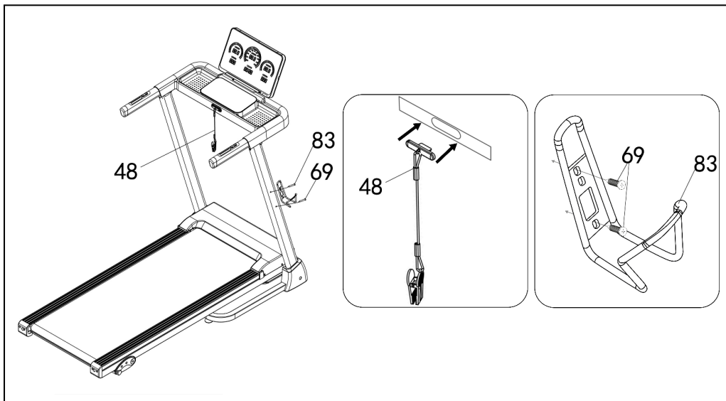
Рисунок 5 — Установка держателя для бутылки
