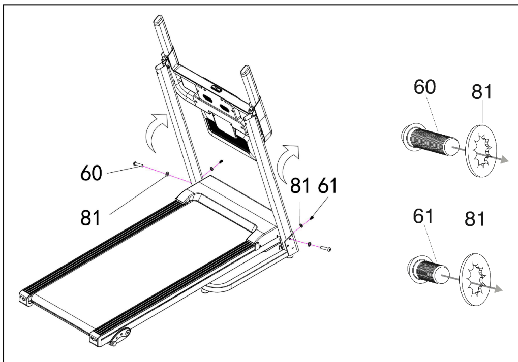
Рисунок 2 — Установка стоек беговой дорожки
