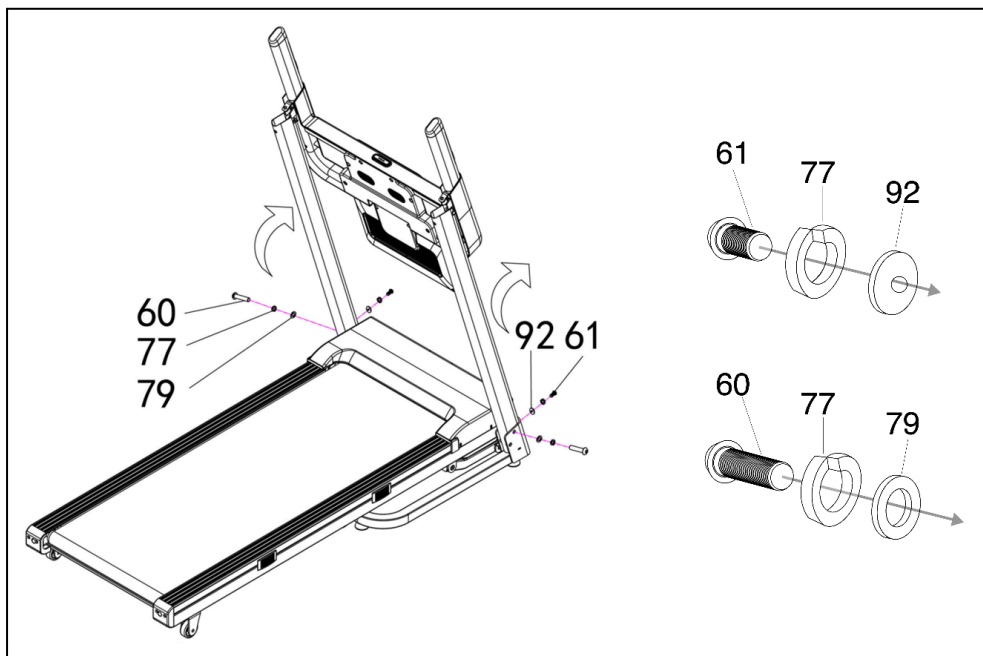
Рисунок 2 — Установка стоек беговой дорожки
