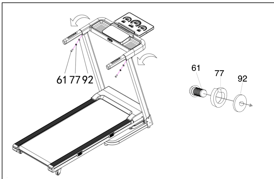
Рисунок 3 — Установка консоли беговой дорожки
