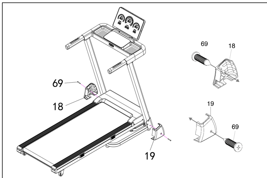
Рисунок 4 — Установка декоративных кожухов
