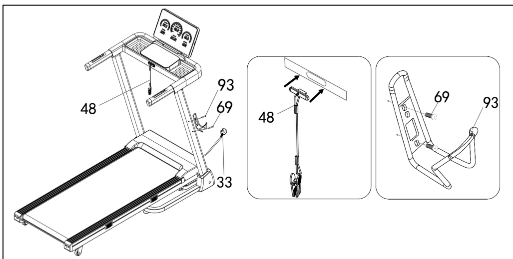
Рисунок 5 — Подключение и запуск беговой дорожки
